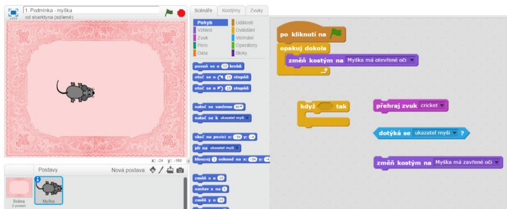
Obrázek 3: Úloha na procvičení používání podmínky
